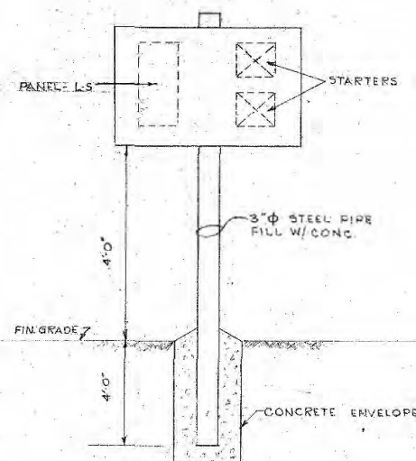
PEDASTAL DETAIL N.T.S.
