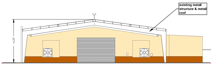
ELEVATION - C
