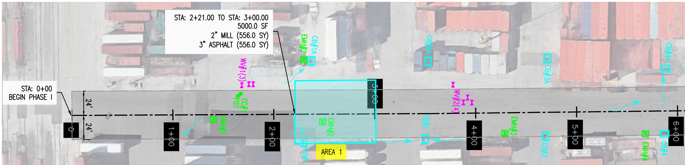
CENTER ROAD STA: 0+00 TO STA: 6+00
